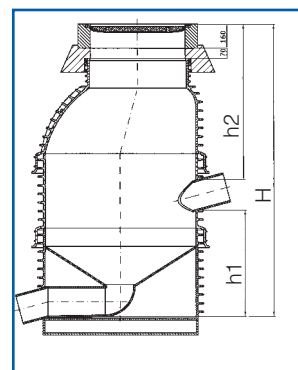
Рис. 43: Вариант- основание + горловина
