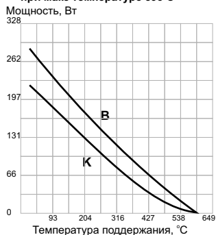
График 4 Максимальные мощности - все кабели с соединением "горячий/холодный" под изоляцией при макс температуре 593°С
