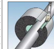
2-Проклеивание шва при помощи клея К 414.
